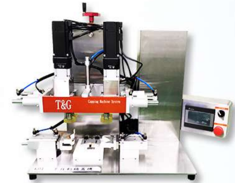
半自動鎖蓋機
